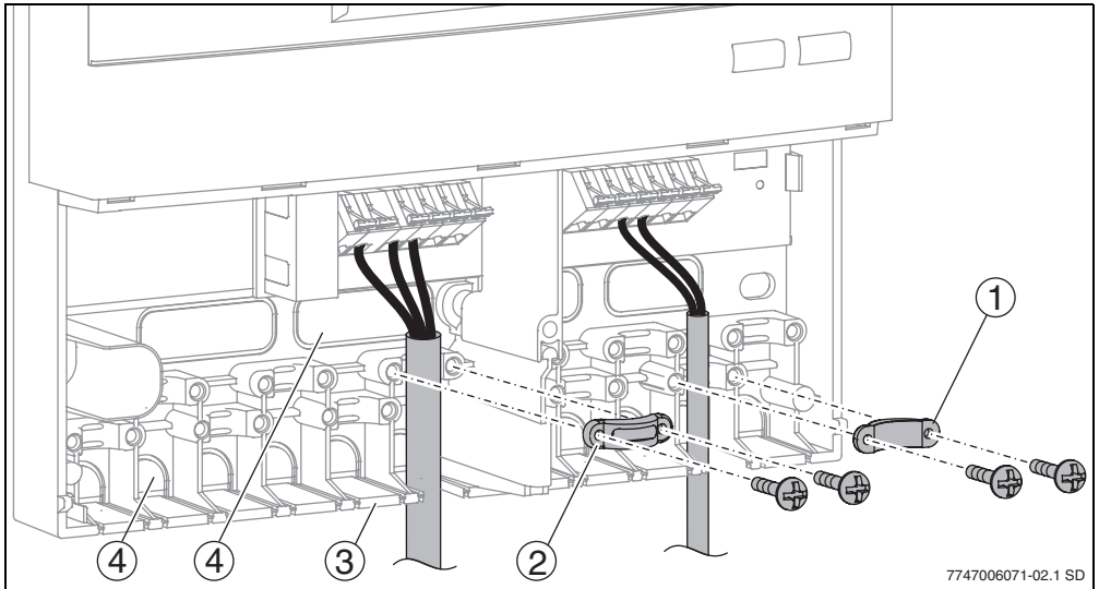
Фиг. 5 Проход и закрепване на кабели
